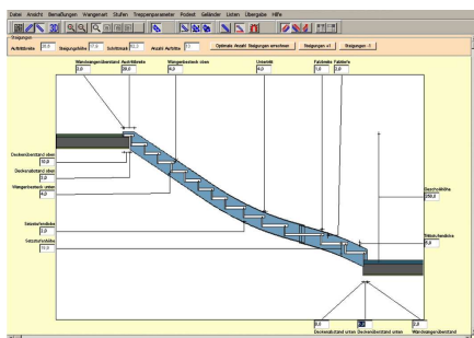
Náhled schodnic u stěny rohových točitých schodů
