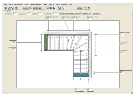
Půdorys rohových točitých schodů
