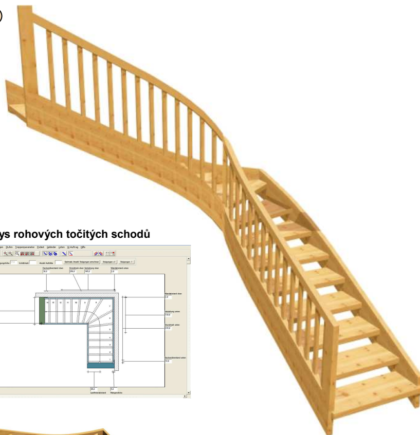
Náhled schodnic u stěny rohových točitých schodů
